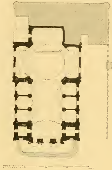
Fig. 9. Ignazkirche zu Klattau. Grundriss.
